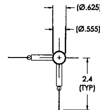
VIEW A-A
