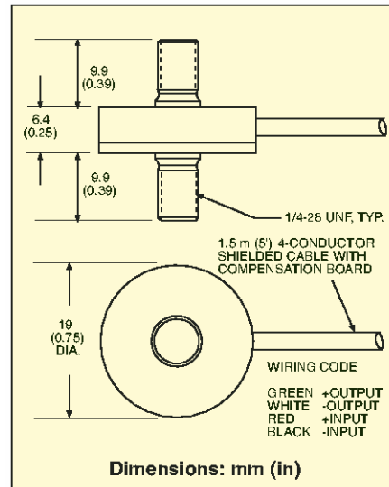
寸法図: 単位 mm(インチ)
